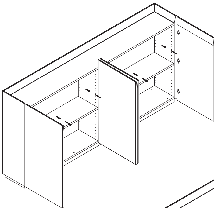
Sideboard Breite / width 2000
