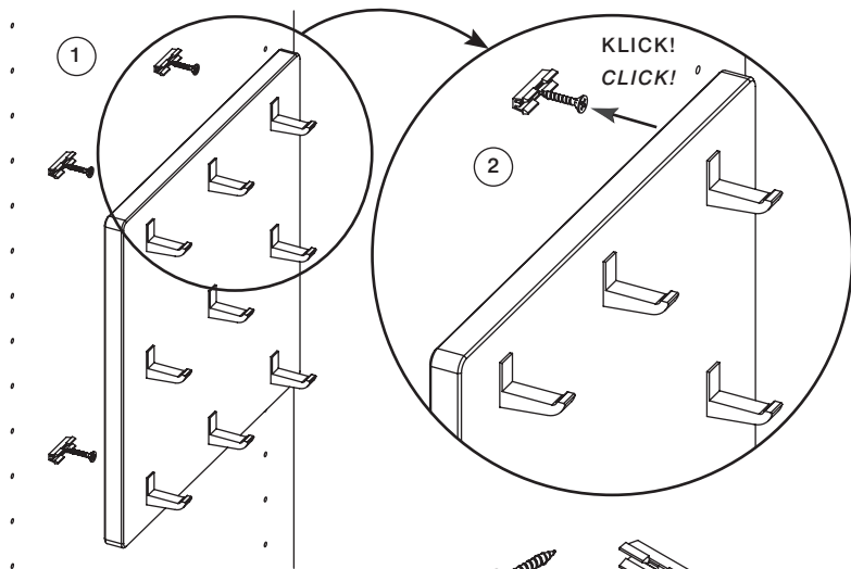
Befestigung an der Möbelseite Mounting on furniture side
