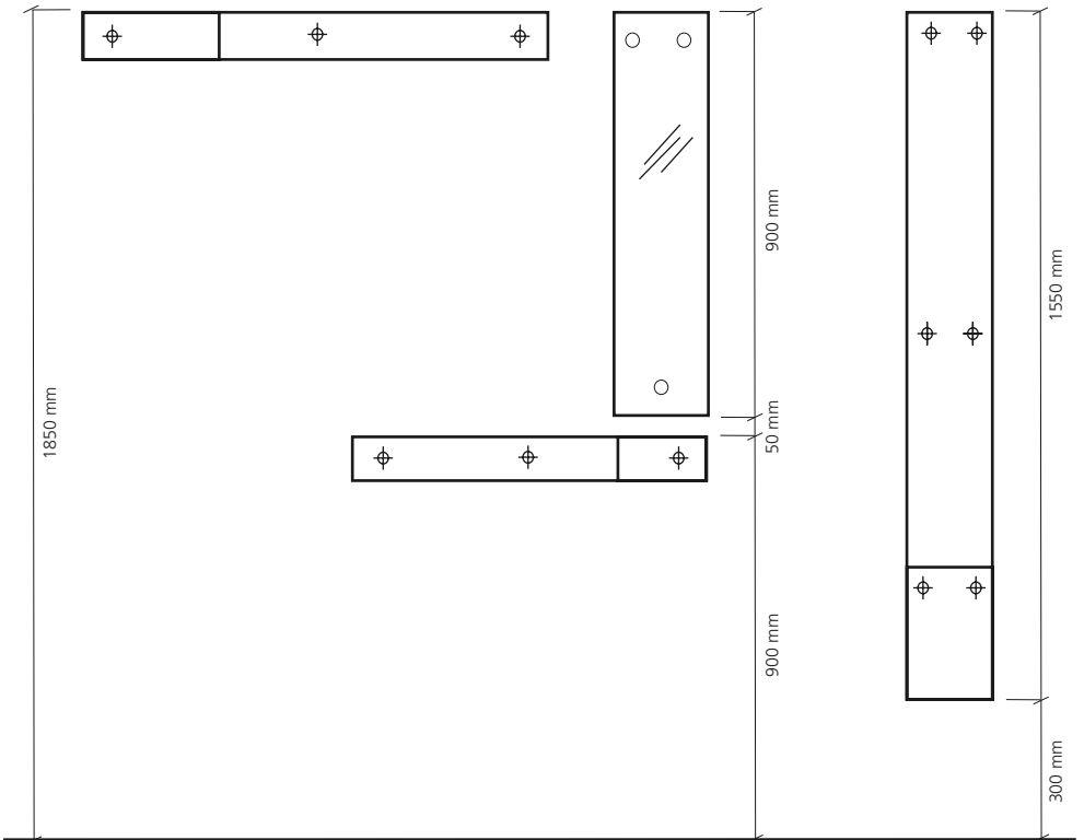
Empfohlene Montagehöhe / Recommended installation height
